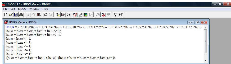
شکل (۳): برنامه خطی نوشته‌شده به زبان لینگو در محیط نرم‌افزار برای انتخاب زیرمجموعه‌ای از دو راهبرد
