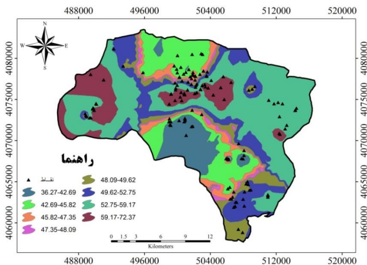
شکل (۷): مقادیر شاخص کیفیت آب‌های زیرزمینی برای مصرف کشاورزی
