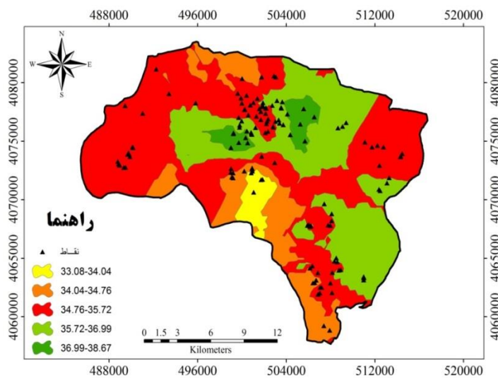
شکل (۶): مقادیر شاخص کیفیت آب‌های زیرزمینی برای مصرف شرب
