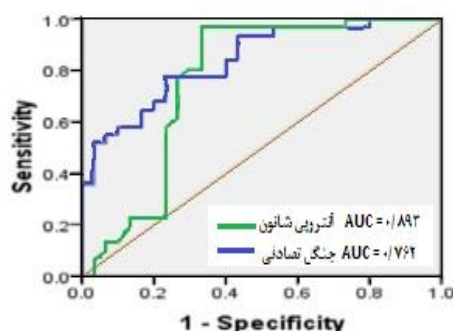
شکل (۵): منحنی ROC و سطح زیر منحنی مربوط به نقشه پتانسیل آب زیرزمینی مدل آنتروپی شانون و جنگل تصادفی Figure (5): ROC curve and area under curve related to groundwater potential map of Entropy and Random forest model
