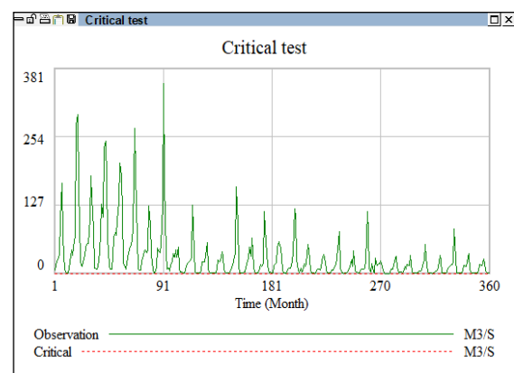
شکل (۴): آزمون شرایط حدی خروجی ایستگاه پل دختر Figure (4): Test of Pol Dokhtar station output critical conditions
