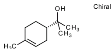
شکل (۱۱): ساختار شیمیایی \alpha -Terpineol
