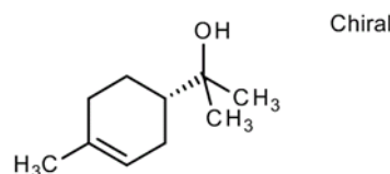
شکل (۱۱): ساختار شیمیایی \alpha -Terpineol Figure (11): Chemical structure of \alpha -Terpineol
