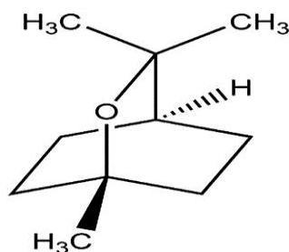
شکل (۱۲): ساختار شیمیایی سینئول 1,8-Cineole Figure (12): Chemical structure of 1,8-Cineole
