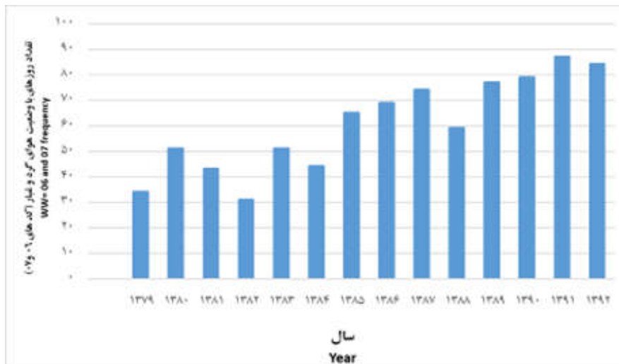
شکل (۴): روزهای دارای طوفان همراه با گردوغبار کدهای ۰۷ و ۰۶ Figure (4): Sand and dust storm Zabol station (WW=07 and 06)
