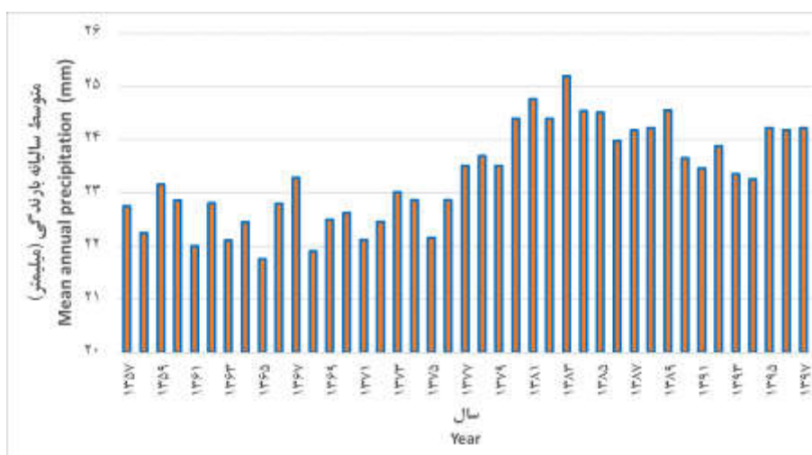
شکل (۶): میانگین سالیانه بارندگی در ایستگاه زابل Figure (6): Mean annual precipitation Zabol station
