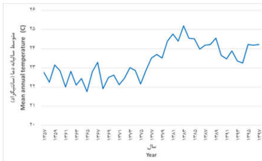
شکل (۵): میانگین سالیانه دما در ایستگاه زابل Figure (5): Mean annual temperature Zabol station
