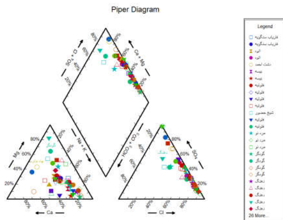
شکل (۶): دیاگرام پایپر دشت فتویه تدرویه
