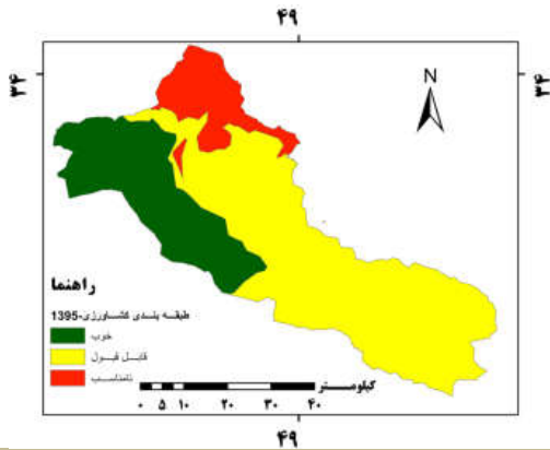
شکل (۹): پهنه بندی کیفیت منابع بر اساس طبقه بندی ویلکاکس Figure (9): Sources quality map based on Wilcox classification
