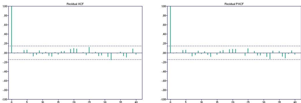
شکل (۵): نمودارهای Residual PACF و Residual ACF در سری داده‌ها پس از پیش‌بینی
