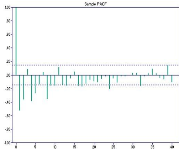
شکل (۳): نمودارهای خودهمبستگی (ACF) و خودهمبستگی جزئی (PACF) در سری داده‌ها
