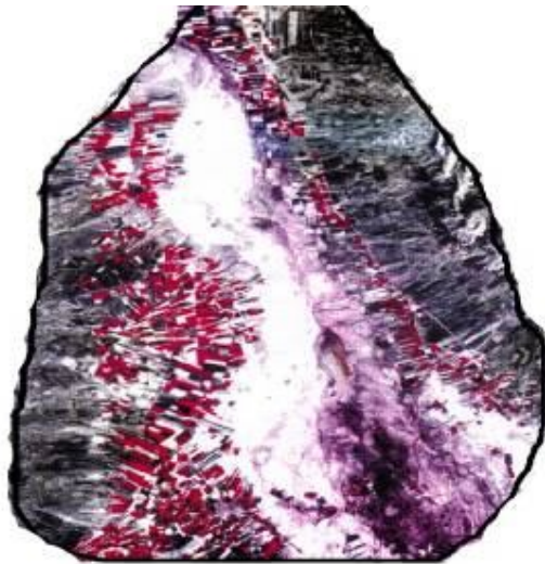
شکل (5): منطقه شورزار در دشت شفاء
