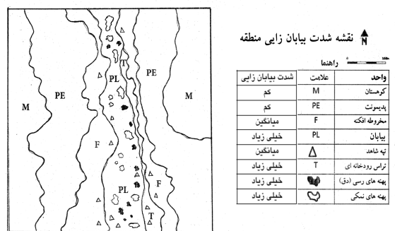
شکل (9): نقشه شدت بیابان‌زایی منطقه مورد مطالعه
