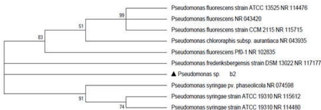
شکل (۲): درخت فیلوژنتیکی ترسیم شده از ژن RNA ریبوزومی 16s جدایه b2 و باکتری های خانواده سودوموناس
