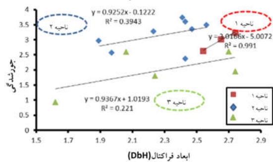
شکل (۵): نمودار تغییرات ابعاد فراکتال در مقابل جورشده‌گی به تفکیک نواحی نمونه‌برداری در آنالیز الک-هیدرومتری
