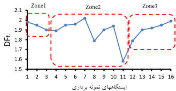
شکل (۱۱): تغییرات مقدار هندسه فراکتال آرایش چگالی فابریک دانه در ایستگاه‌های نمونه‌برداری شده لس‌های گلستان
