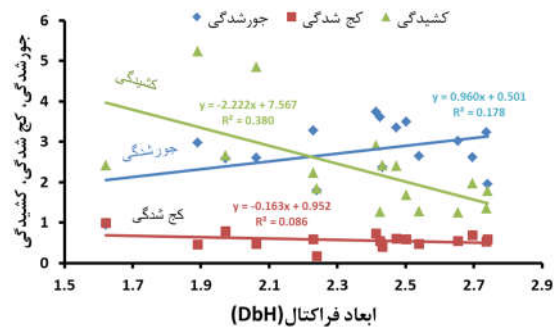
شکل (۶): تغییرات جورشده‌گی، کج‌شدگی، کشیدگی را در مقابل ابعاد فراکتال در آنالیز الک-هیدرومتری
