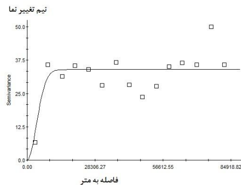
شکل (۷): واریوگرام تجربی برای مقادیر سیلت (silt)
