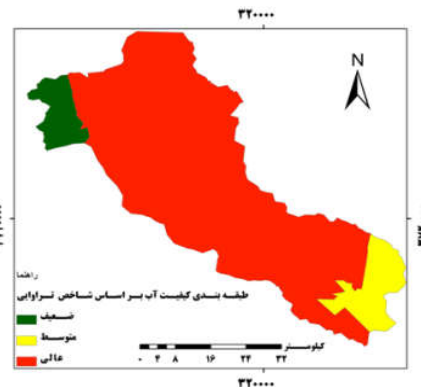
شکل (۵): طبقه‌بندی کیفیت منابع زیرزمینی بر اساس شاخص تراوایی
