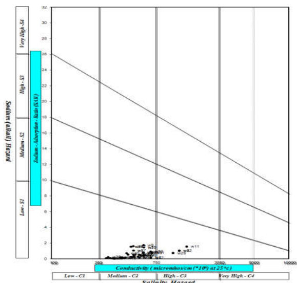
شکل (۷): دیاگرام ویلکاکس برای سال ۱۳۹۵
