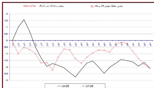
شکل (۲): نمودار من-کندال مربوط پارامتر EC Figure (2): Mann-Kendal graph for EC
