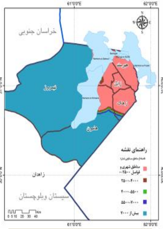
شکل (۱۰): نقشه طبقه‌بندی شده فاصله از مناطق مسکونی Figure (10): Distance classified map from residential areas
