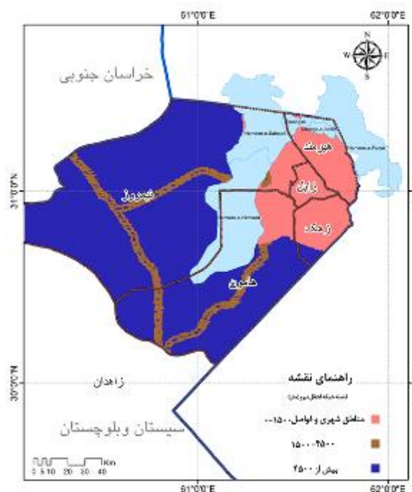
شکل (۸): نقشه طبقه‌بندی شده نزدیکی به شبکه انتقال نیرو Figure (8): Distance classified map to the power transmission network
