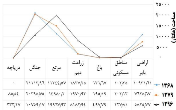
شکل (۴): مساحت طبقات مختلف کاربری اراضی در طی سال های مختلف مورد بررسی Figure (4): Area of different classes of land use during different years
