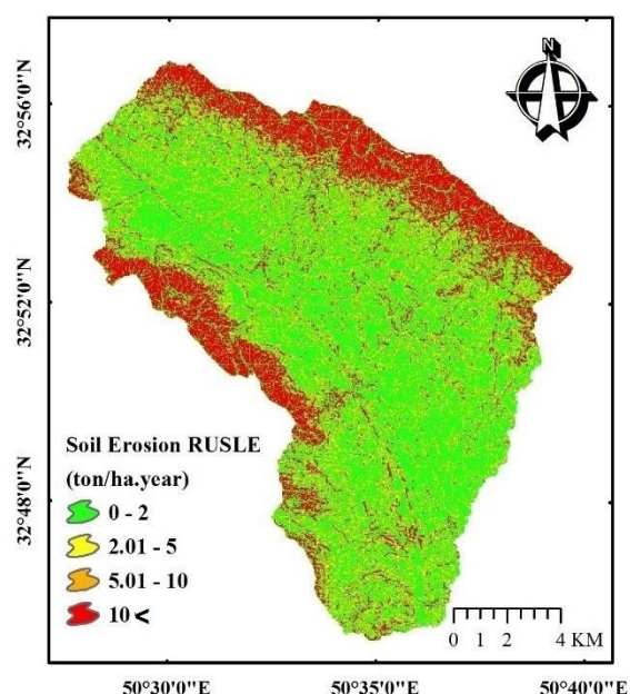
شکل (۴): فرسایش سالانه خاک بر اساس مدل RUSLE Figure (4): Annual soil erosion based on RUSLE model
