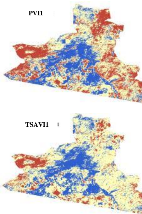
شکل (۳): ترکیب آزمون من-کندال و شیب تیل سن شاخص‌های طیفی. مناطق با رنگ قرمز دارای روند کاهشی معنی دار و مناطق با رنگ آبی دارای روند افزایشی معنادار است. مناطق زردرنگ روند تغییرات معناداری ندارند. Figure (3): Combination of the Me-Kendal test and the tilt slope of the Spectral Indicators
