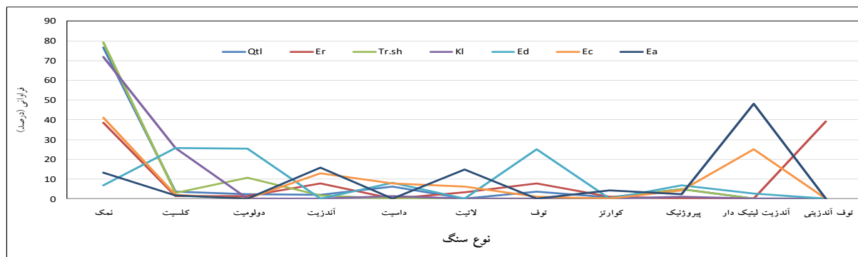
شکل (۲): متوسط فراوانی سنگ‌ها در واحدهای مختلف زمین‌شناسی حوضه با تحلیل مورفوسکوپی نمونه‌ها Figure (2): The average frequency of rocks in different geologic units of watershed using morphoscopic analysis of samples
