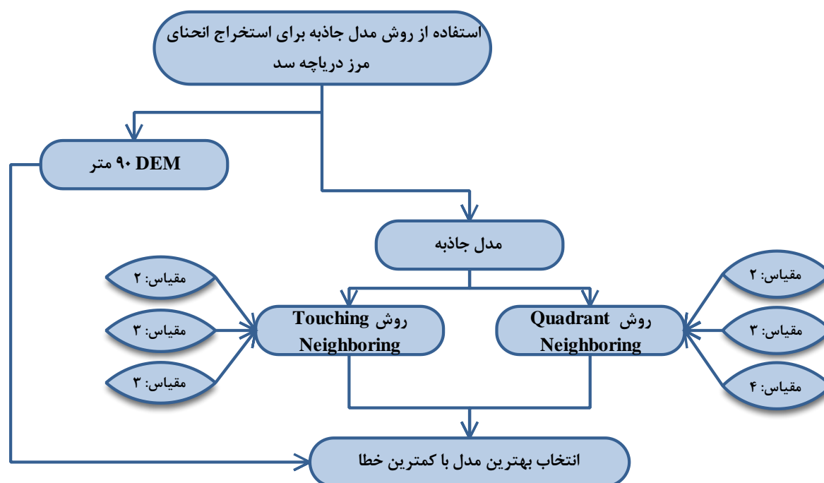
شکل (۳): مراحل مختلف تحقیق به منظور افزایش قدرت تفکیک مکانی مدل رقومی ارتفاع (DEM) با استفاده از الگوریتم جاذبه برای بررسی انحناى دریاچه سد کوثر
