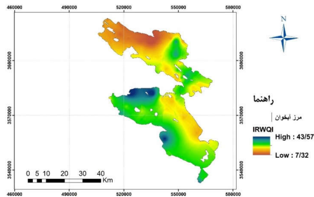
شکل (۹): نقشه پهنه‌بندی IRWQI در آبخوان‌های لنجان‌نجدآباد
