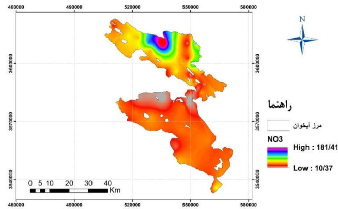
شکل (۸): نقشه پهنه‌بندی نترات در آبخوان‌های لنجان‌نجدآباد
