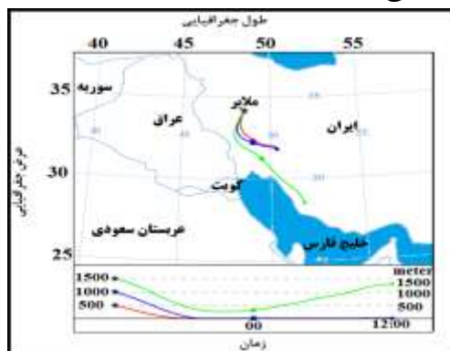
شکل (۷): مسیر ورود ذرات گردوغبار به ملایر
