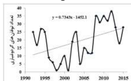
شکل (۲): روند سالانه طوفان‌های گردوغبار در ملایر Figure (2): Trend of annual dust storm in Malayer
