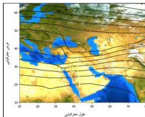
شکل (۵): الگوی مولد گردوغبار در تراز ۵۰۰ هکتوپاسکال
