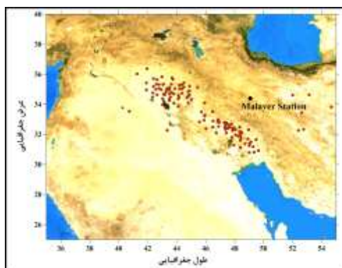
شکل (۸): سرچشمه های گردوغبار ورودی به ملایر
