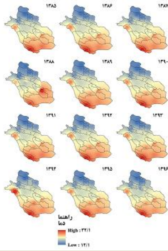
شکل (۵): روند تغییرات شاخص دما (سانتی‌گراد) در بازه زمانی ۱۳۸۵ تا ۱۳۹۶ Figure (5): The trend of changes in temperature index (°C) for the period 2006-2017
