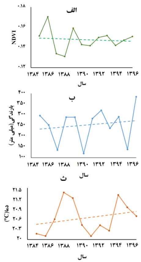
شکل (۶): الف. روند تغییرات شاخص‌های NDVI؛ ب. بارندگی (میلی‌متر)؛ ج. دما (سانتی‌گراد) در بازه زمانی ۲۰۰۶-۲۰۱۷ Figure (6): the trend of changes of indices A) NDVI; b) rainfall (mm) and c) temperature (°C) for the period of 2006-2017
