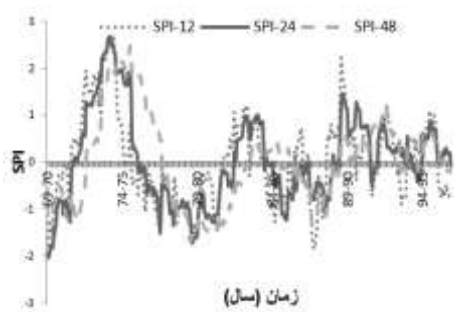
شکل (۲): روند تغییرات شاخص SPI در حوضه دشت سلماس در طول دوره آماری ۱۳۶۹-۱۳۷۰ تا ۱۳۹۵-۱۳۹۶
