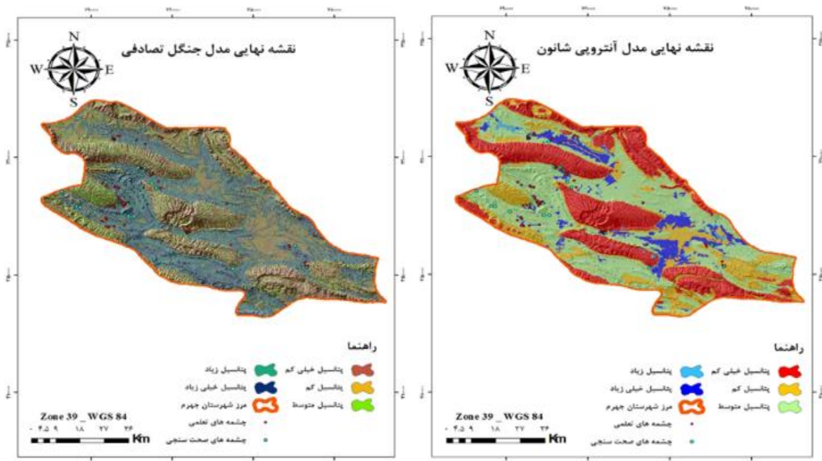
شکل (۴): نقشه نهایی پتانسیل آب زیرزمینی منطقه مورد مطالعه مدل آنتروپی شانون (راست) و جنگل تصادفی (چپ)
